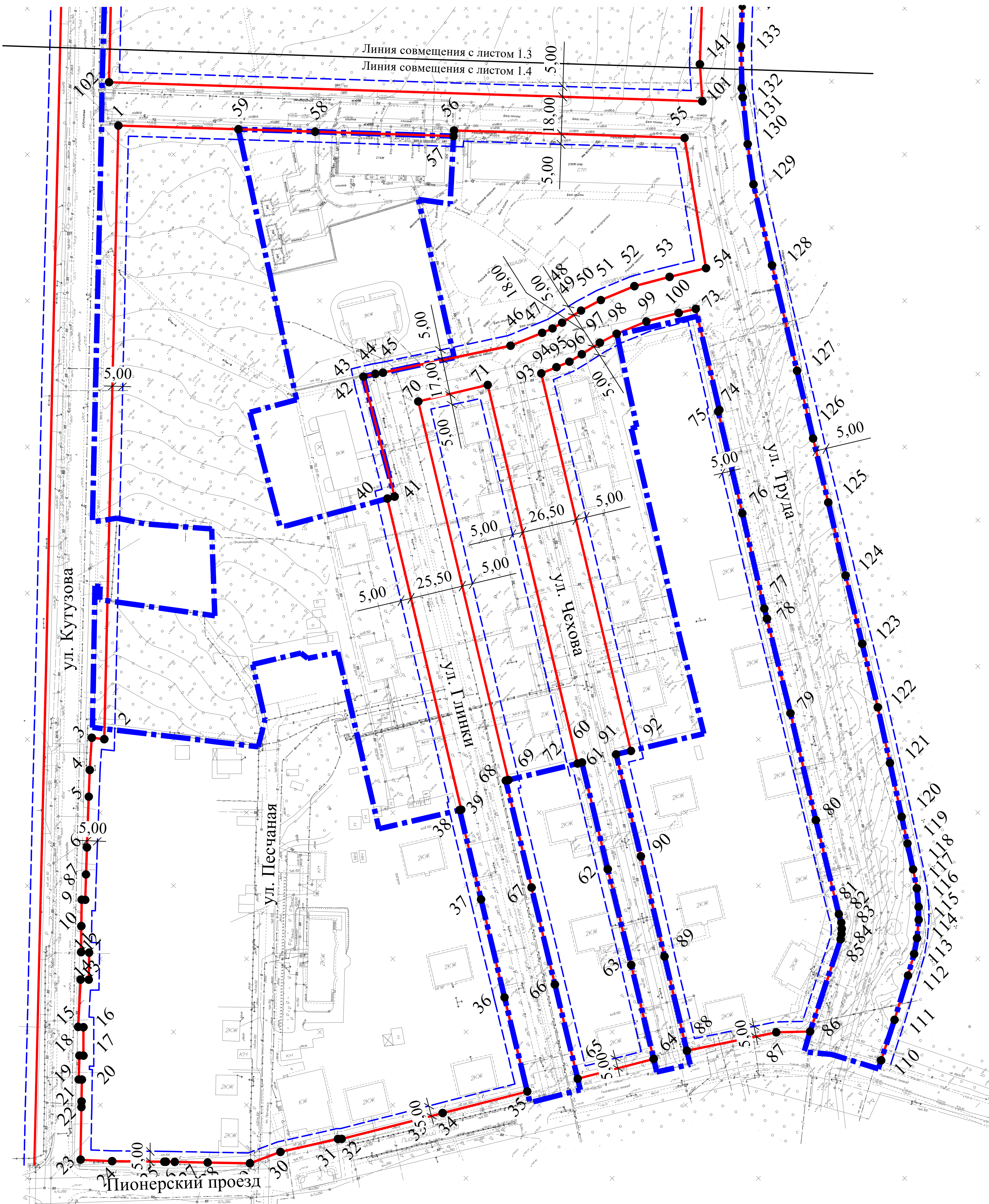
Чертеж красных линий М 1:1000
