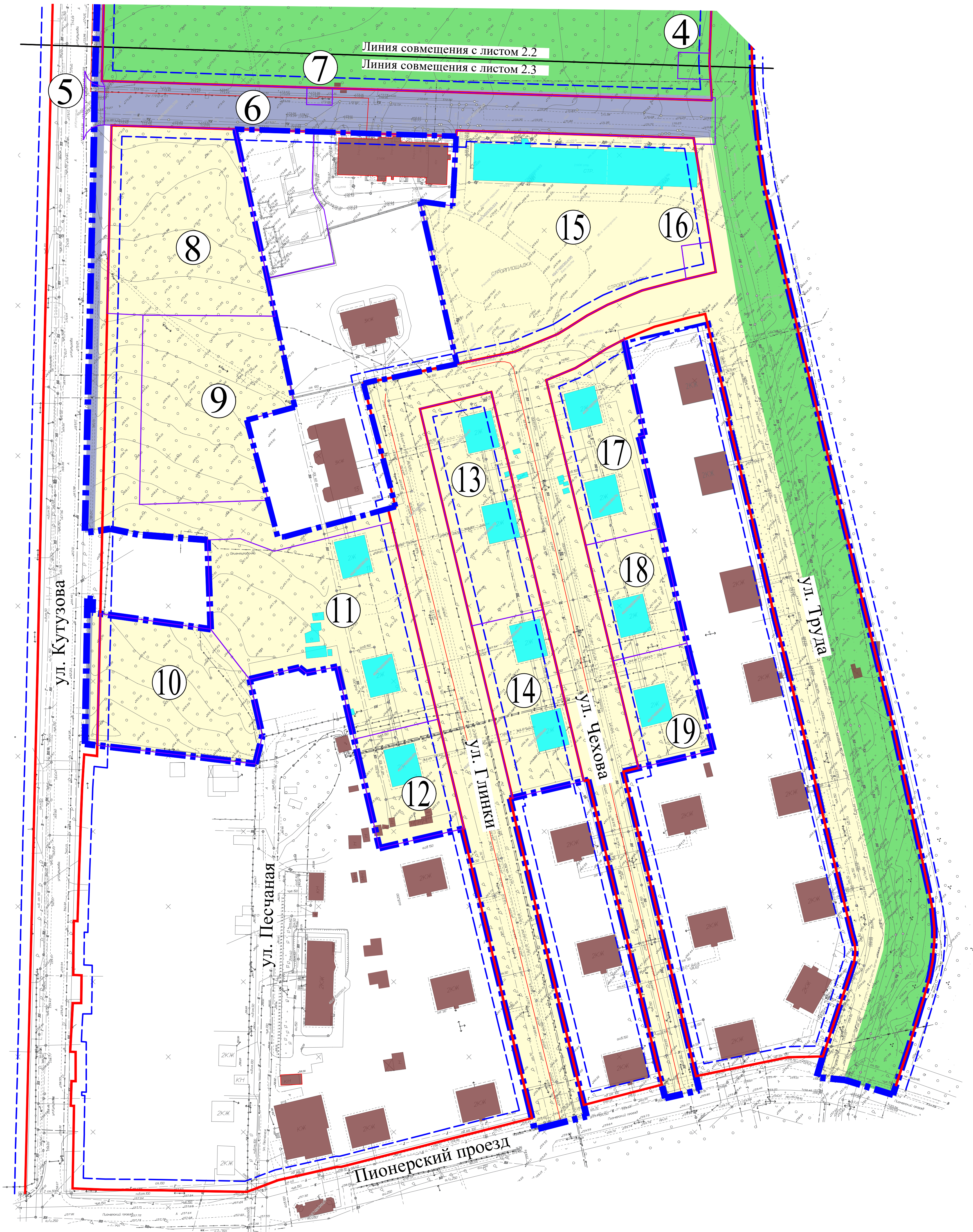
Схема, отображающая местоположение существующих объектов капитального строительства М 1:1000
