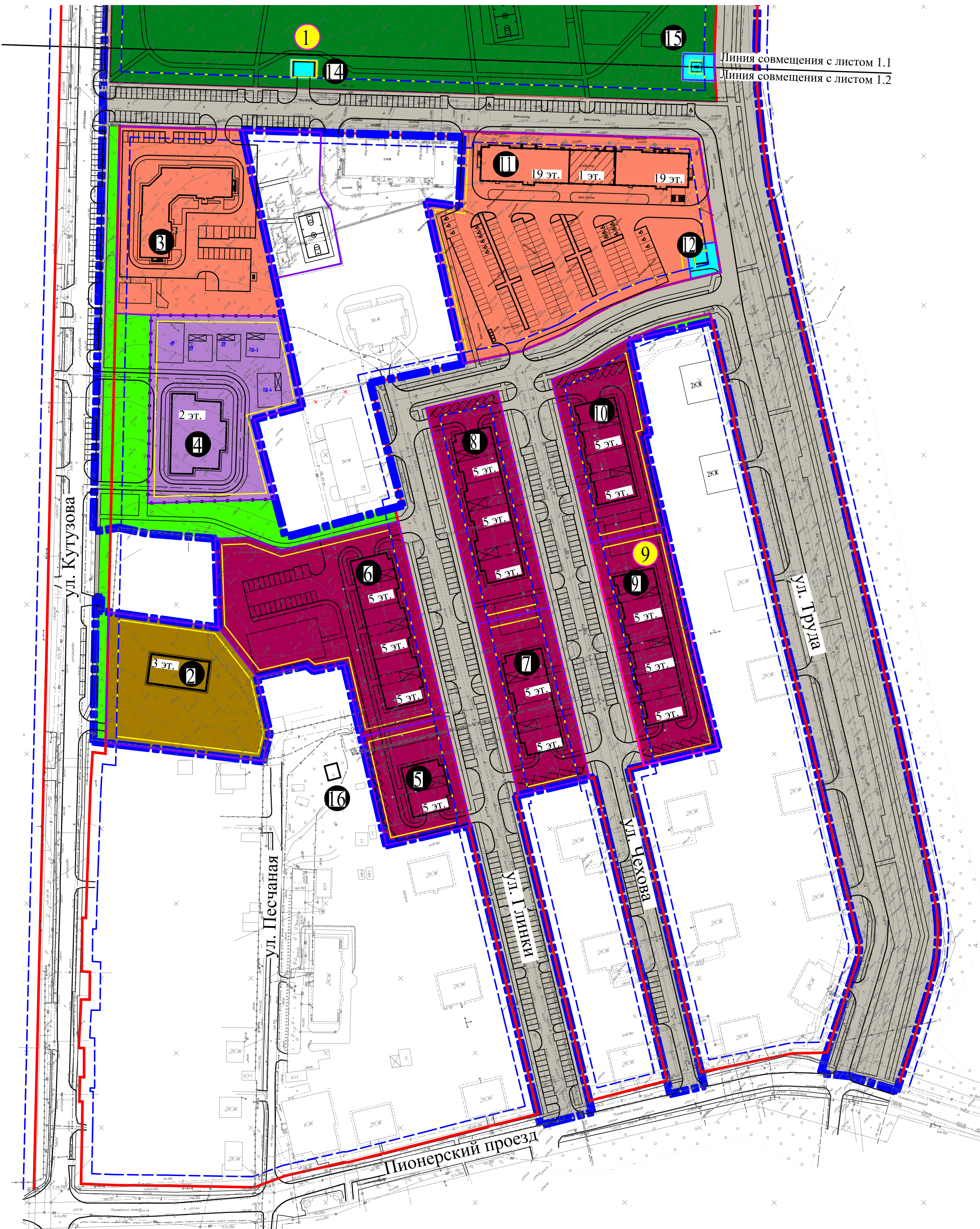
Чертеж планировки территории М 1:1000
