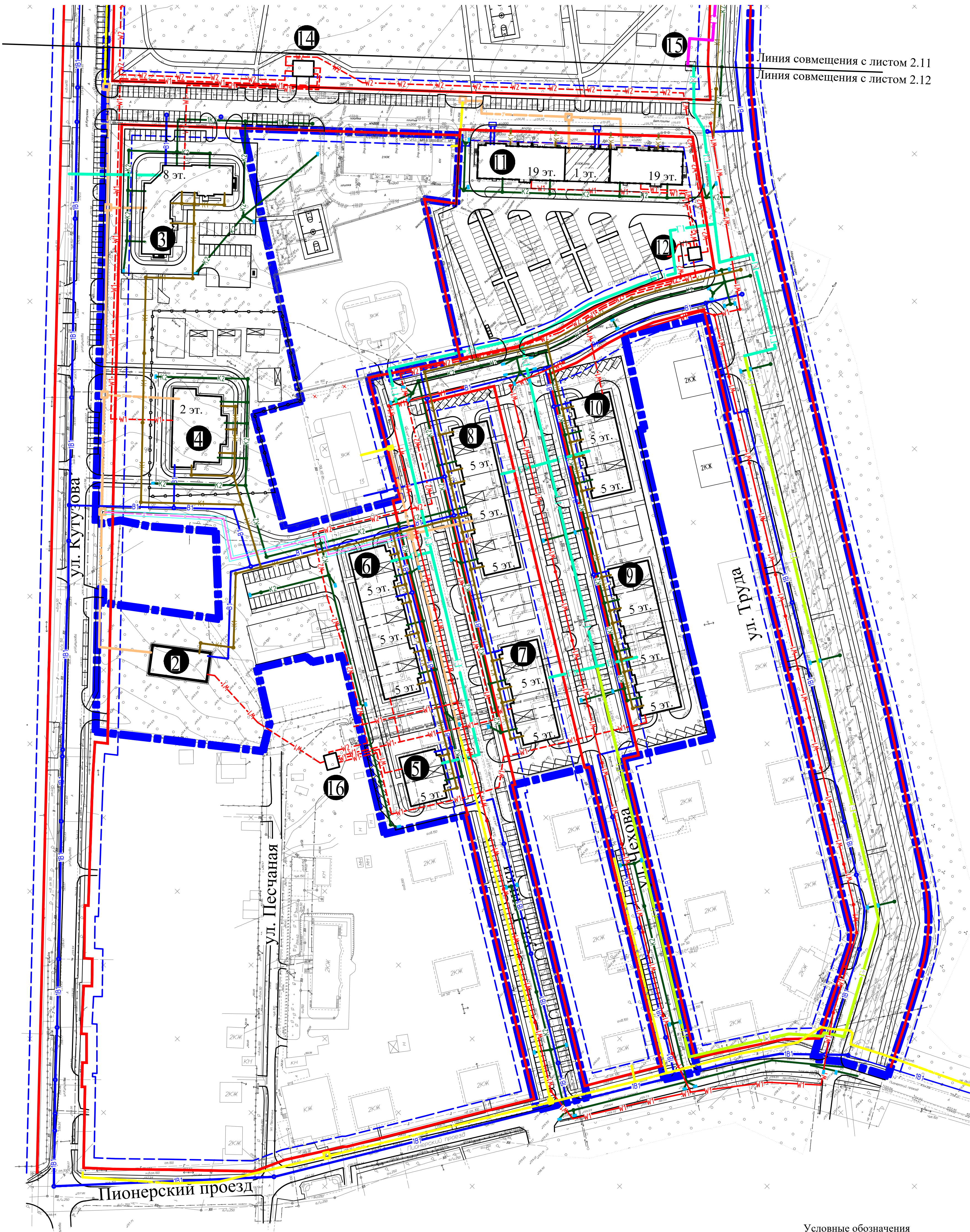
Схема размещения инженерных сетей и сооружений М 1:1000
