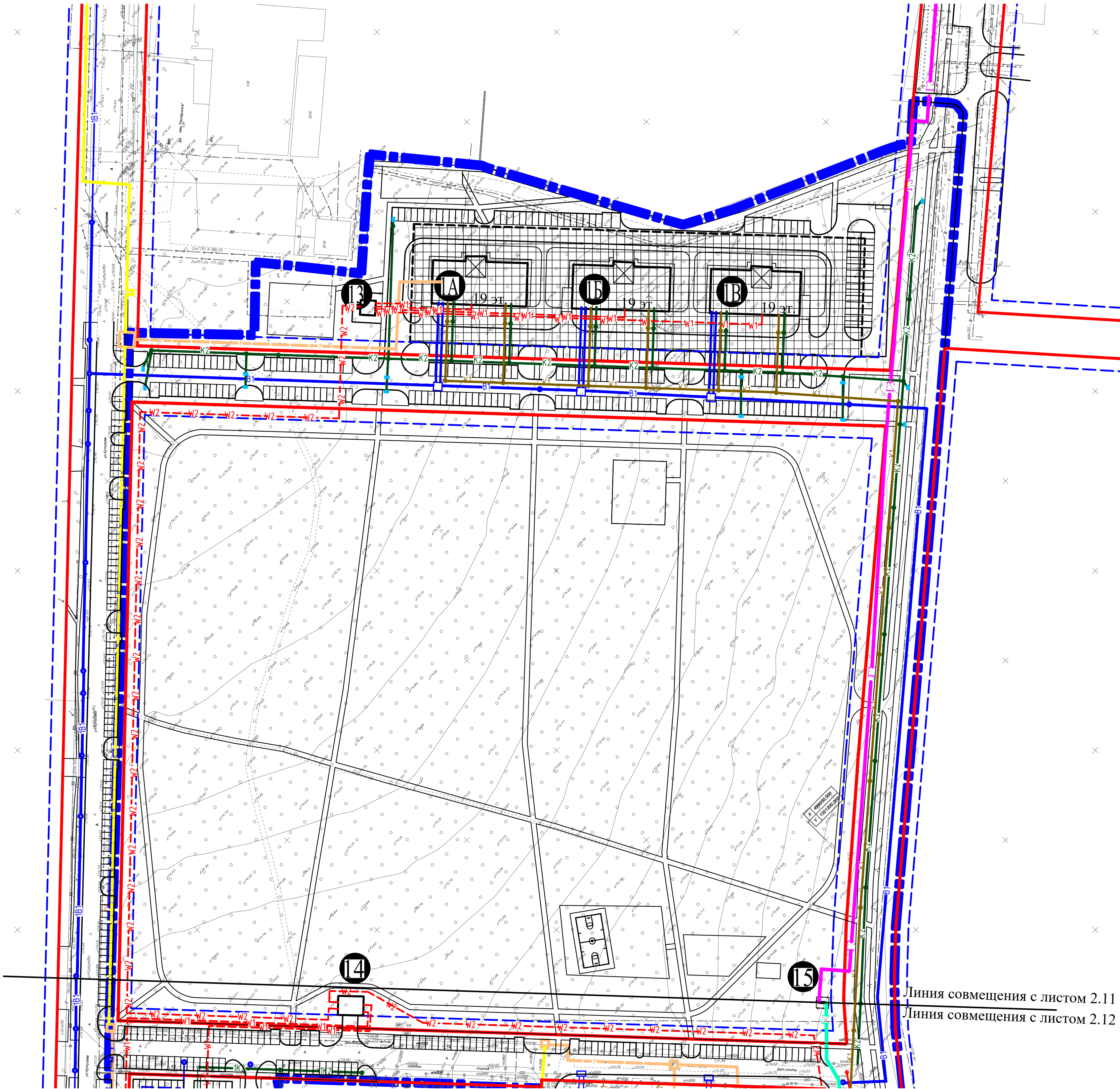
Схема размещения инженерных сетей и сооружений М 1:1000
